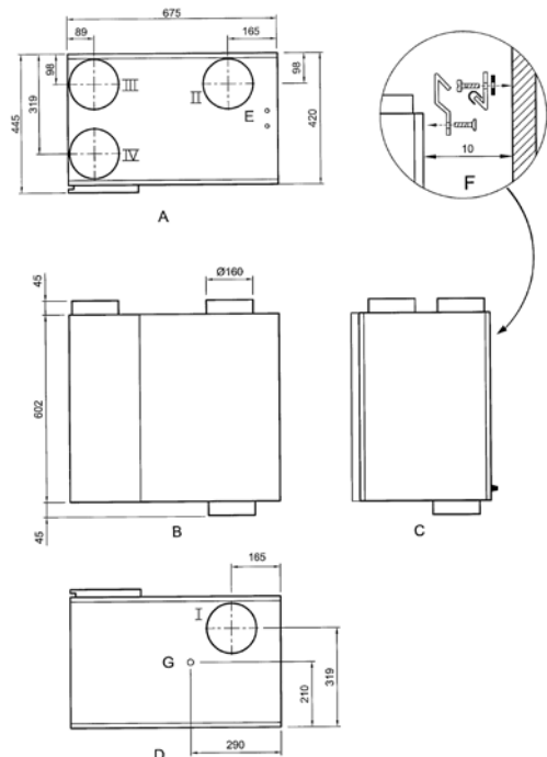
Fig. 12: Geroteerde Renovent HR325 met 3-boven/1-onder aansluiting
