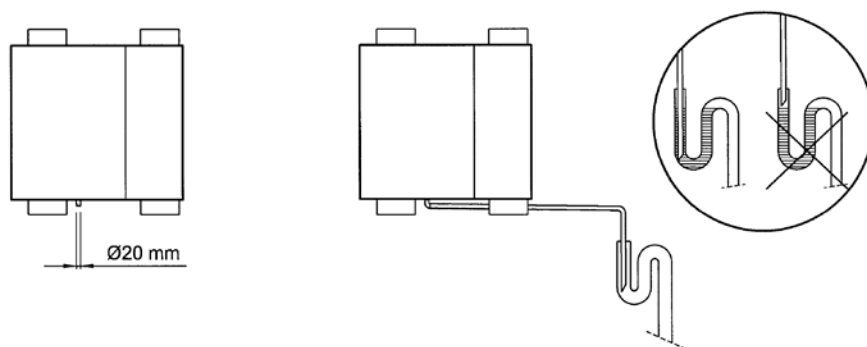
Figuur 5: Aansluiting Renovent HR 325 op binnenriolering.
