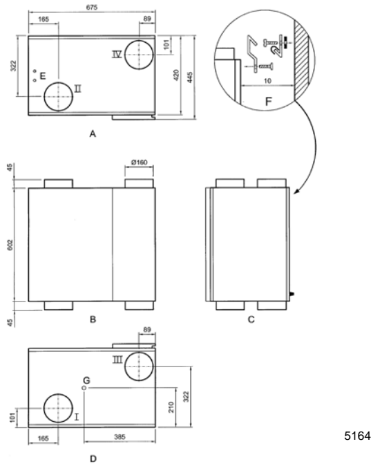
Figuur 7: Renovent HR 325 met b/o aansluitingen.
