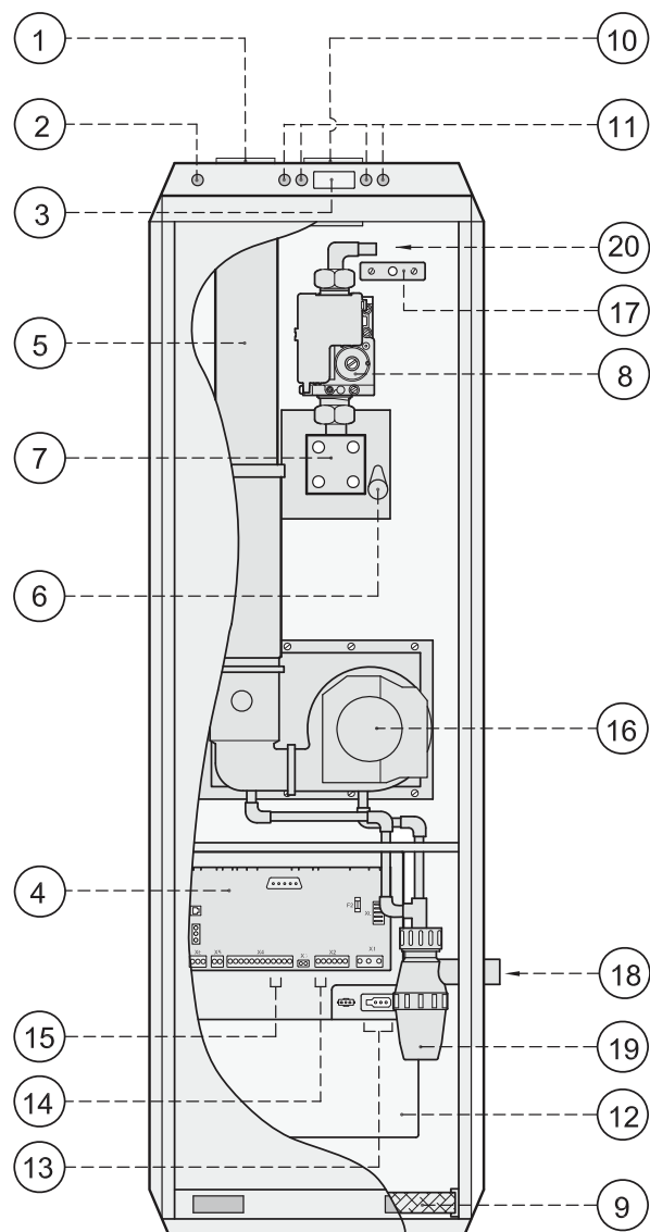
Upflow-uitvoering
