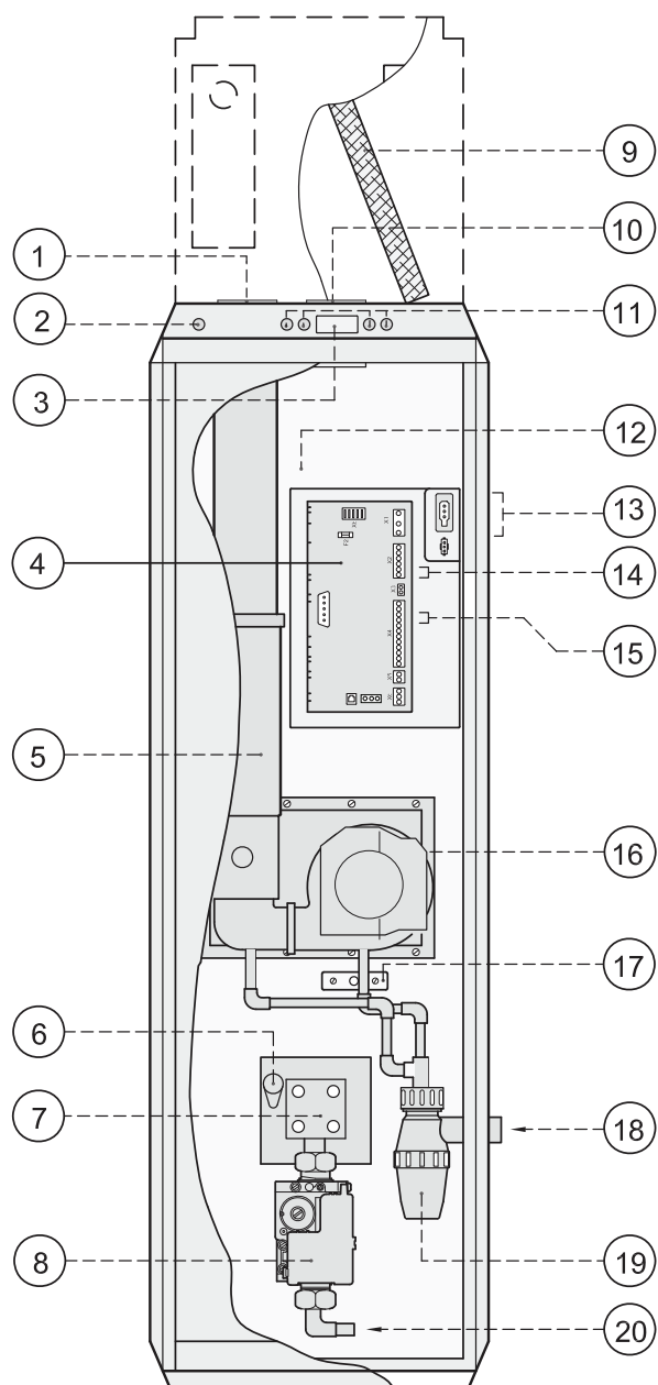
Downflow-uitvoering
