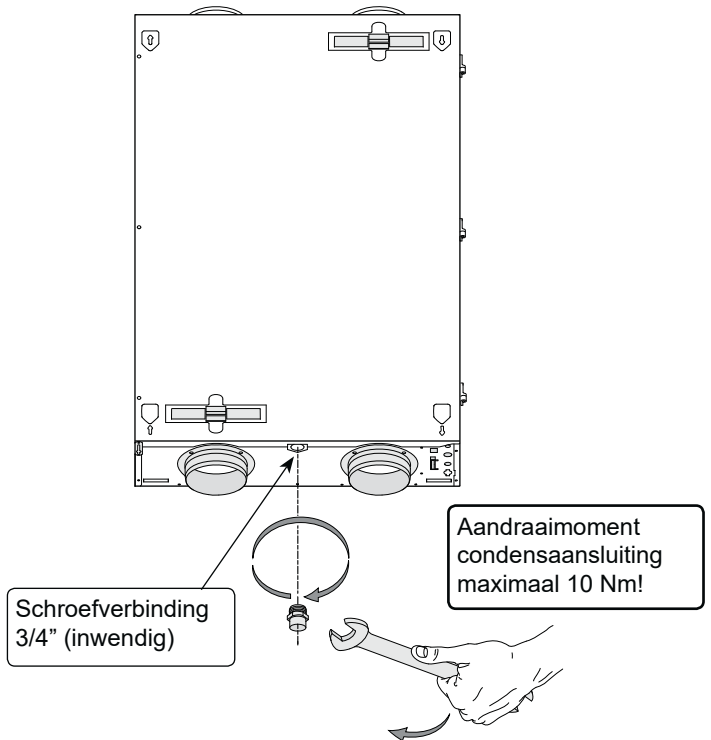
Montage condensafvoer aansluiting in CWL - F - 150 Excellent (VHZ)
