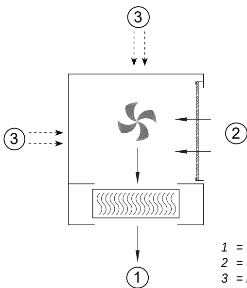
Downflow-Ausführung
