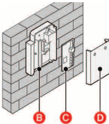
Wandmontage (optioneel)
