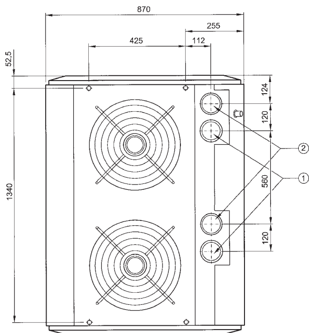
Figuur 7: Ophangpunten B-80 IGX en B-92 IGX
