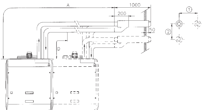
Figuur 15: Horizontale toe- en afvoersysteem Flair IGX.
