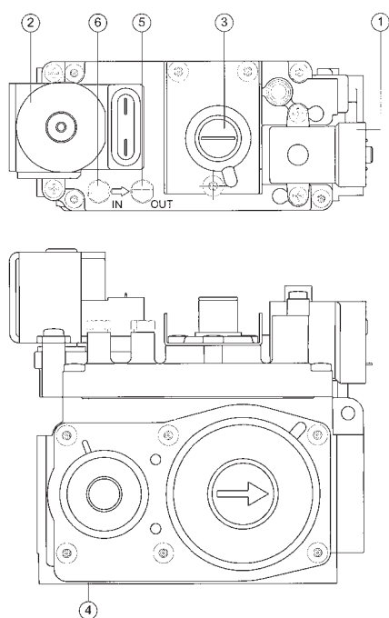
Figuur 19: Beveiligingsafsluiter
