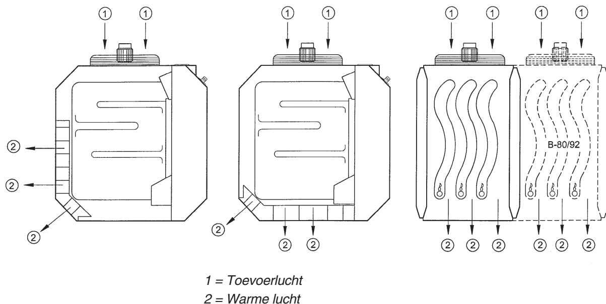
Figuur 2: Principeschets Flair-serie Luchtzijdig
