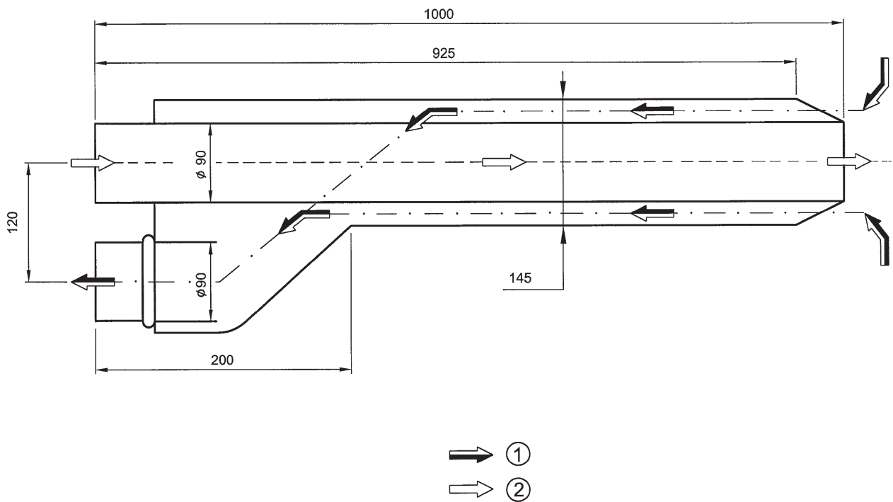
Figuur 12: Horizontale doorvoer \varnothing 80
