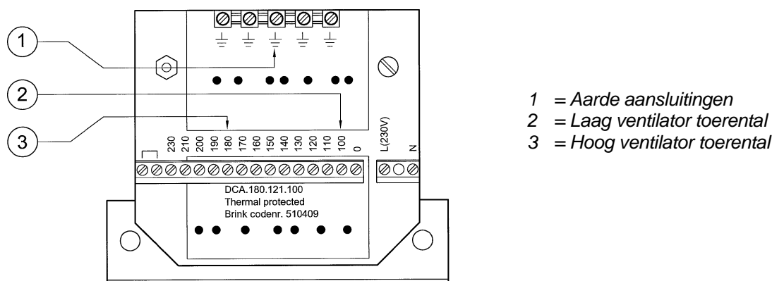
Figuur 5. Regeltransformator.
