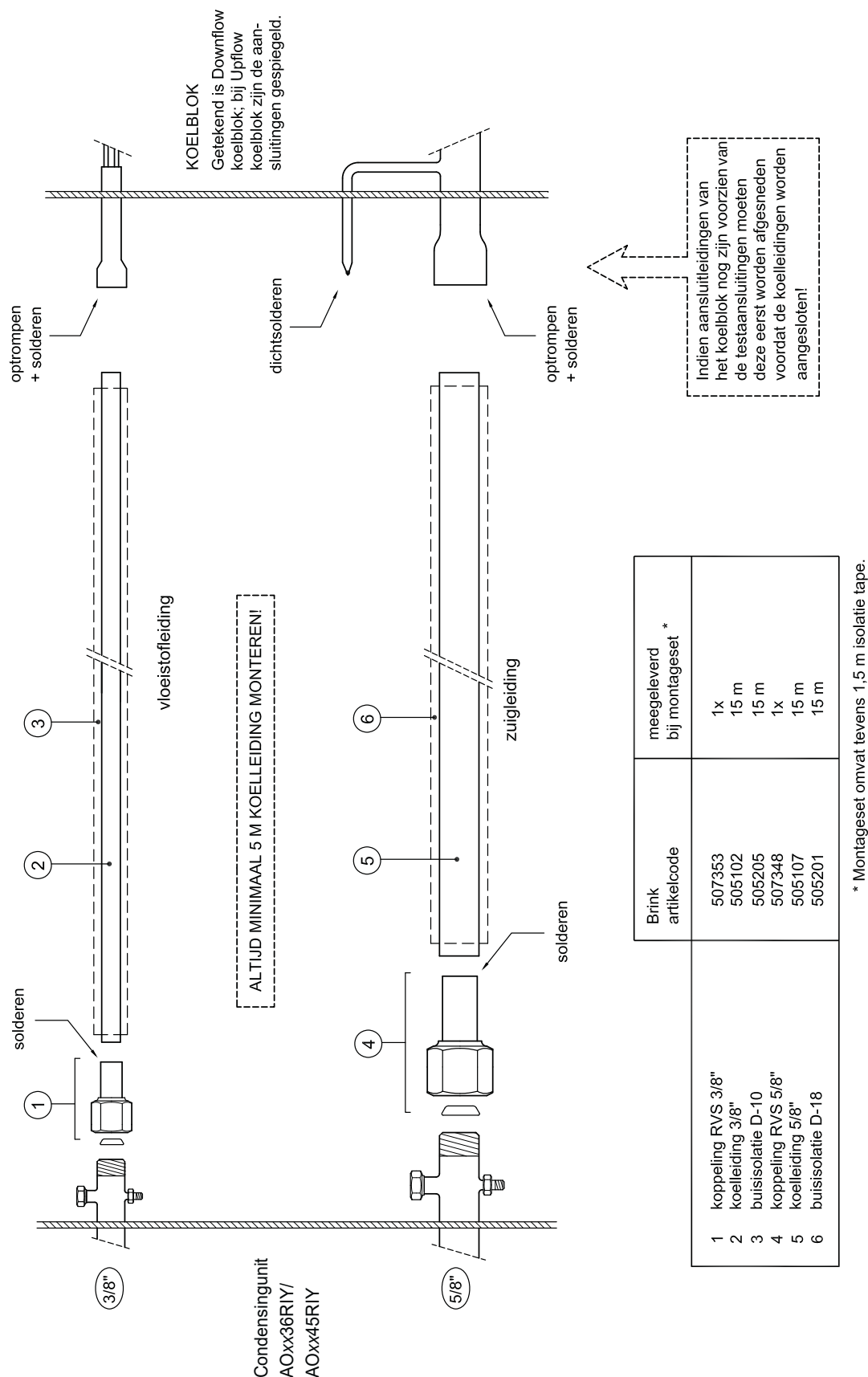
Leidingschema koeling met combinatie B1/B2, combinatie C1/C2, combinatie D1/D2, combinatie E1/E2, combinatie G & combinatie H met condensingunit AOxx36RIY(F) & AOxx45RIY(F)
