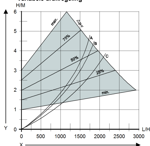
Variable drukregeling
