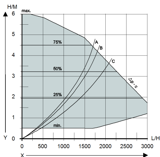
Constante drukregeling
