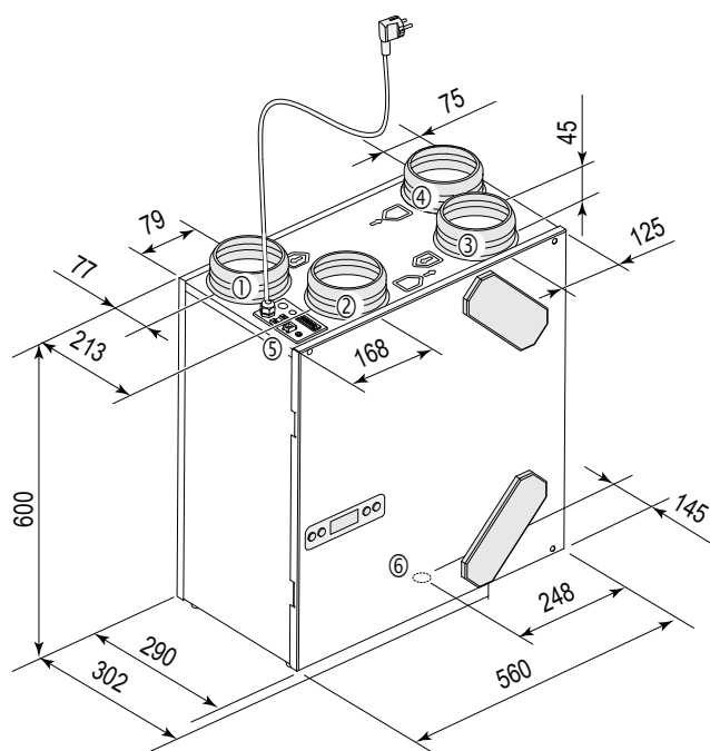
Renovent Excellent 180 a la derecha 4/0
