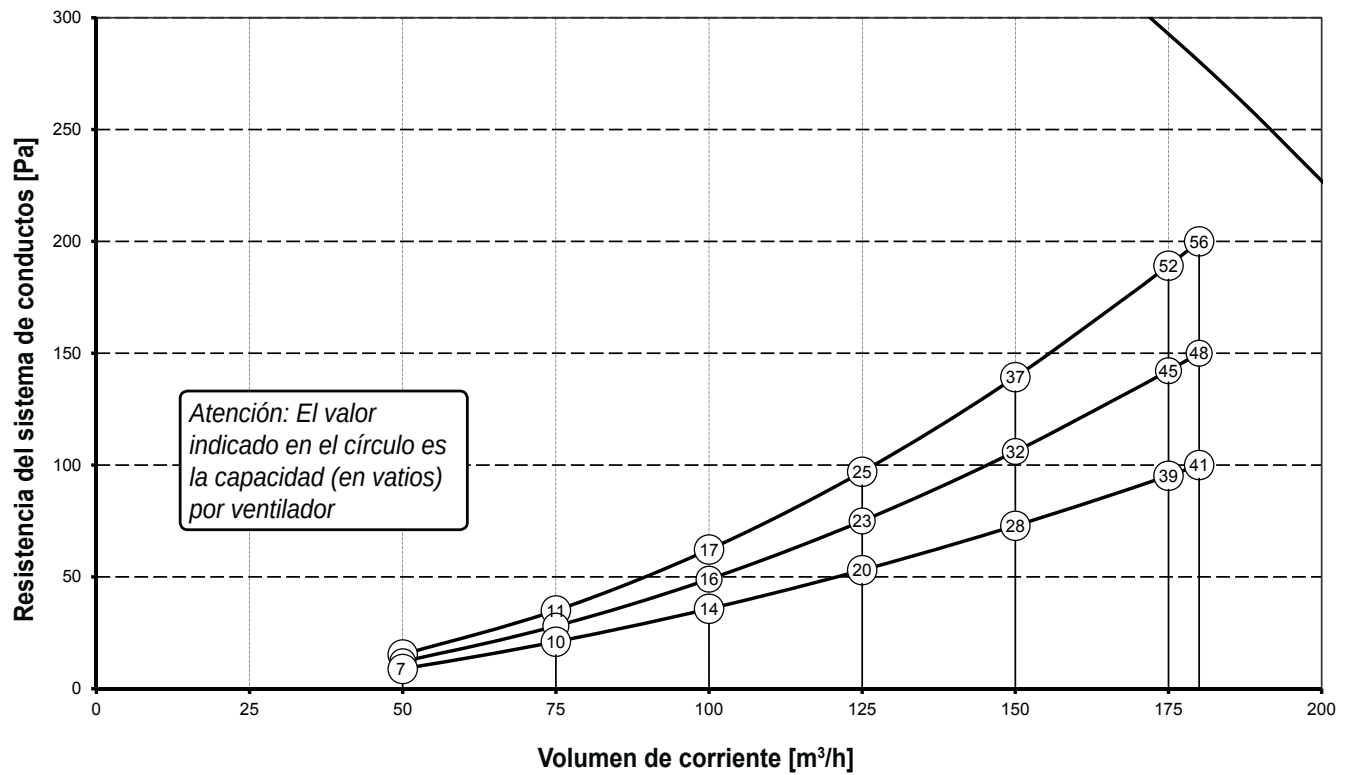
Gráfico del ventilador Renovent Excellent 180
