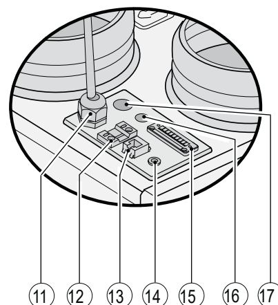
Conexiones parte superior del equipo
