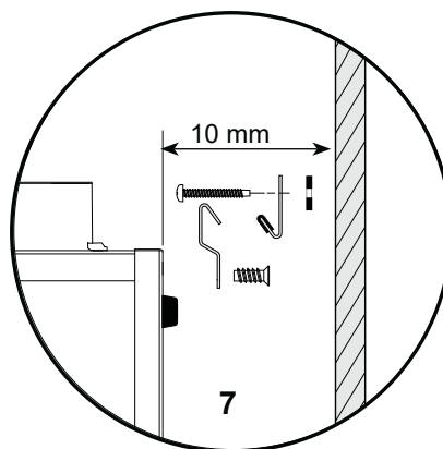
Montaža pribora za pritrditev na steno
