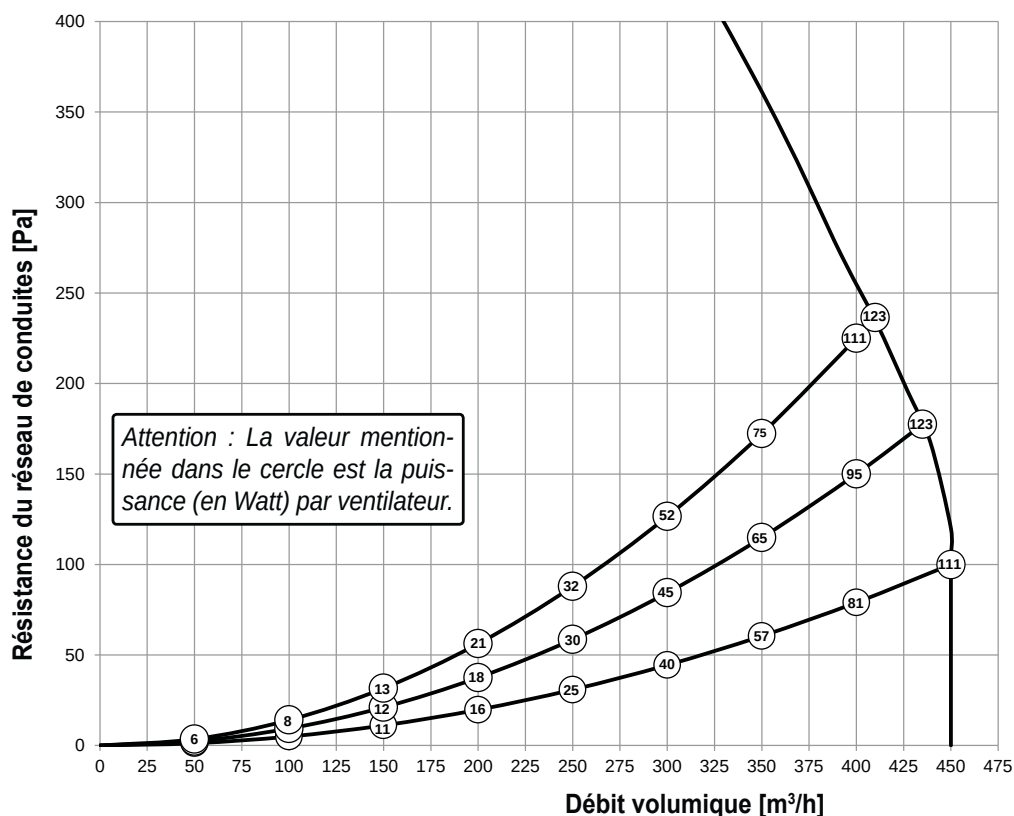
Graphique du ventilateur du Renovent Excellent 450
