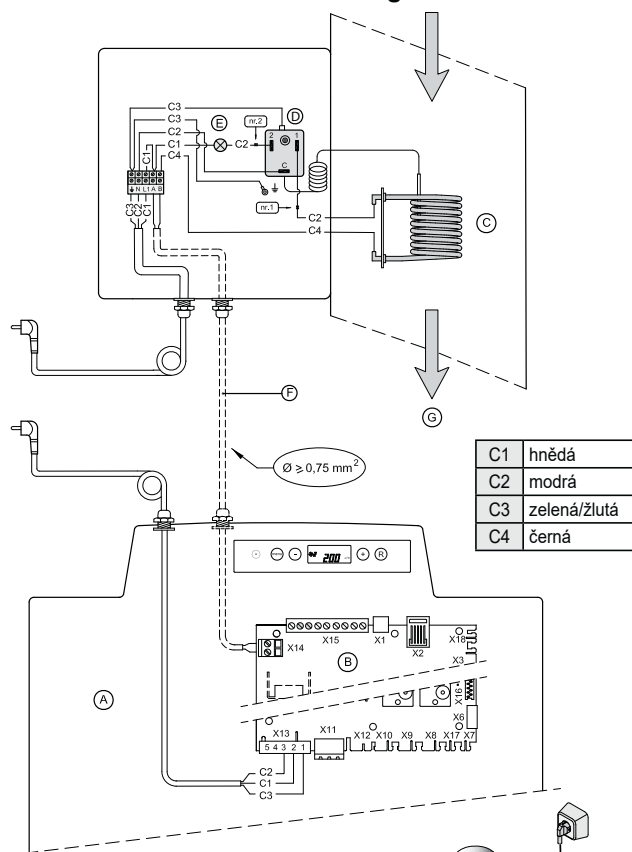
Předehřívací registr navíc
