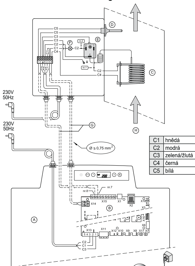
Dohřívací registr
