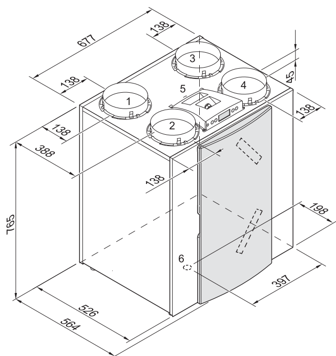
Renovent Excellent 450 pravostranné vyhotovení 4/0
