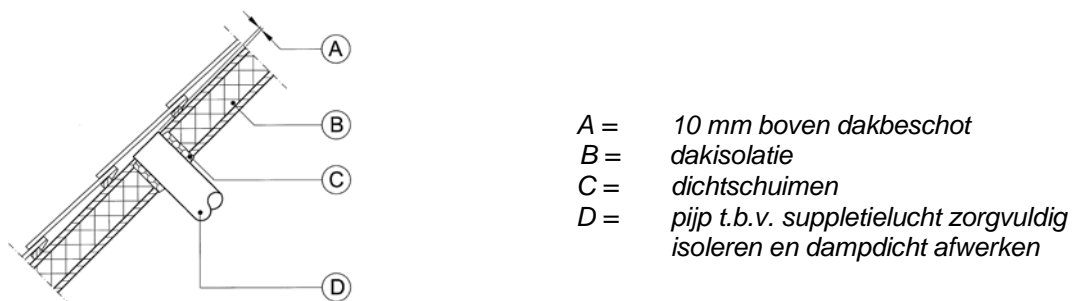
Figuur 3: Doorvoer buitenluchtkanal door het dakbeschoot onder de pannen.
