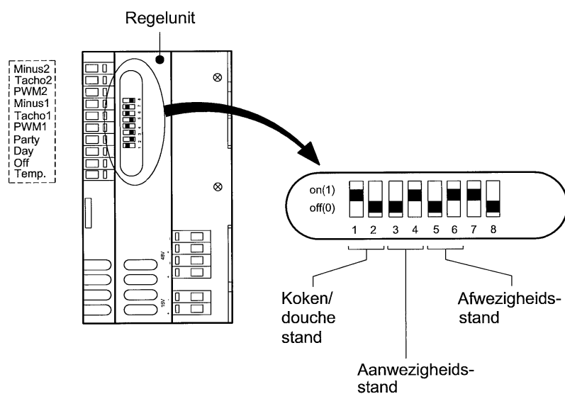
Figuur 13 Vooraanzicht regelunit.
