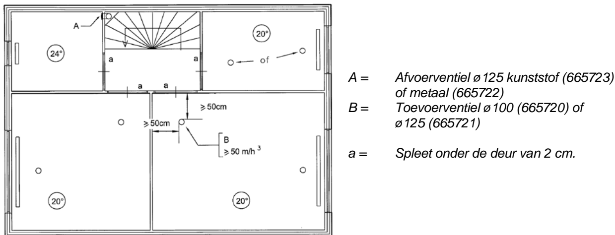
Figuur 4: Plaatsing afvoer- en toevoerventilen.
