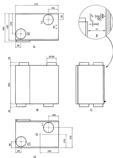
Figuur 10: Renovent HR 325 met b/o aansluitingen.
