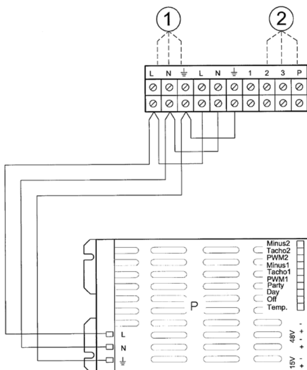
Figuur 6: Elektrische aansluitingen op regelunit.
