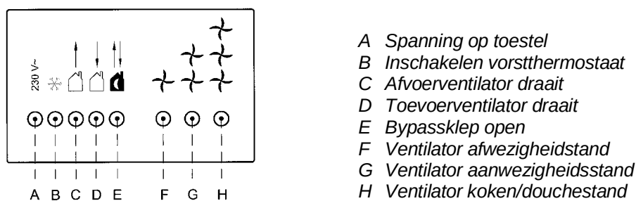
Figuur 9: Aanzicht LED-paneel
