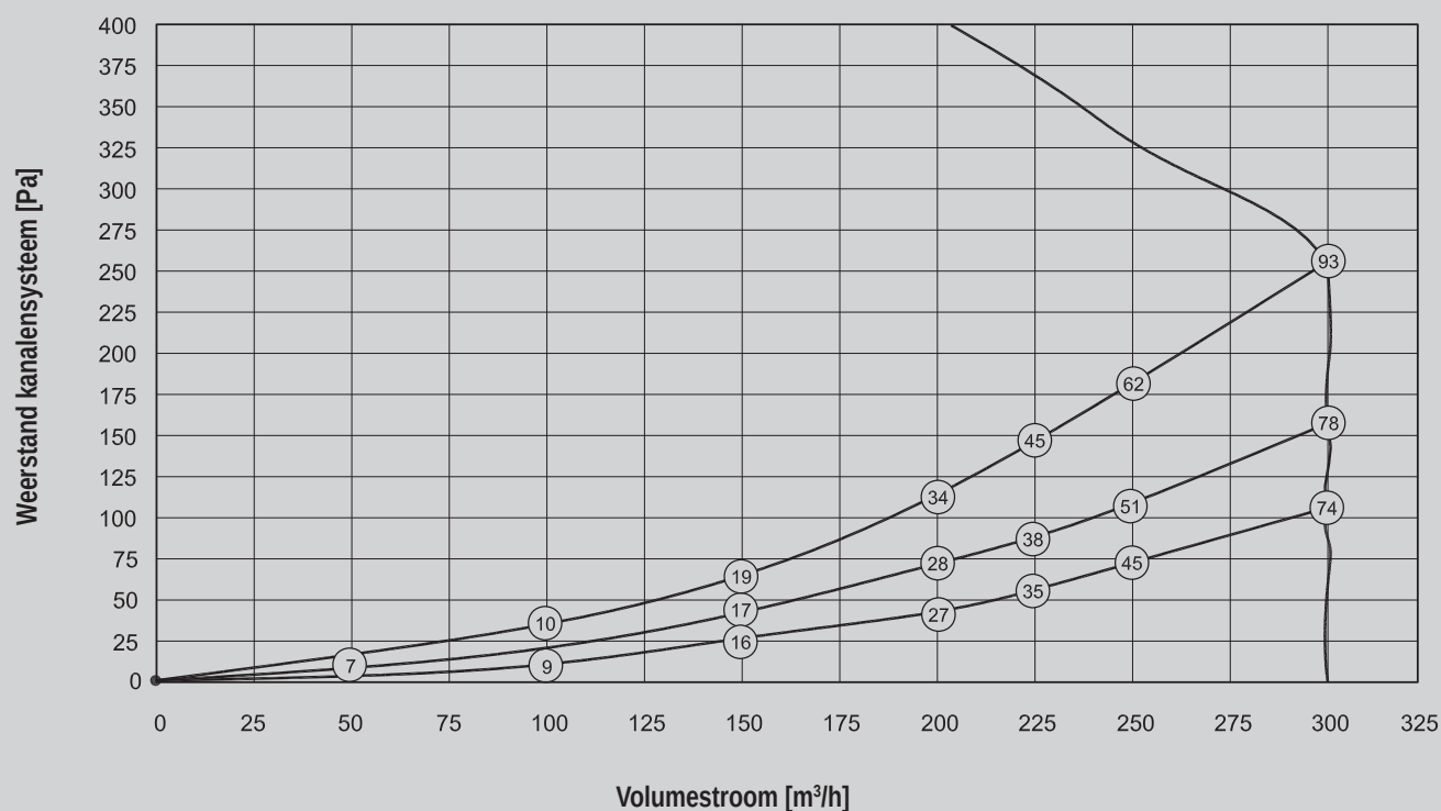
Ventilatorgrafiek Renovent HR Medium
