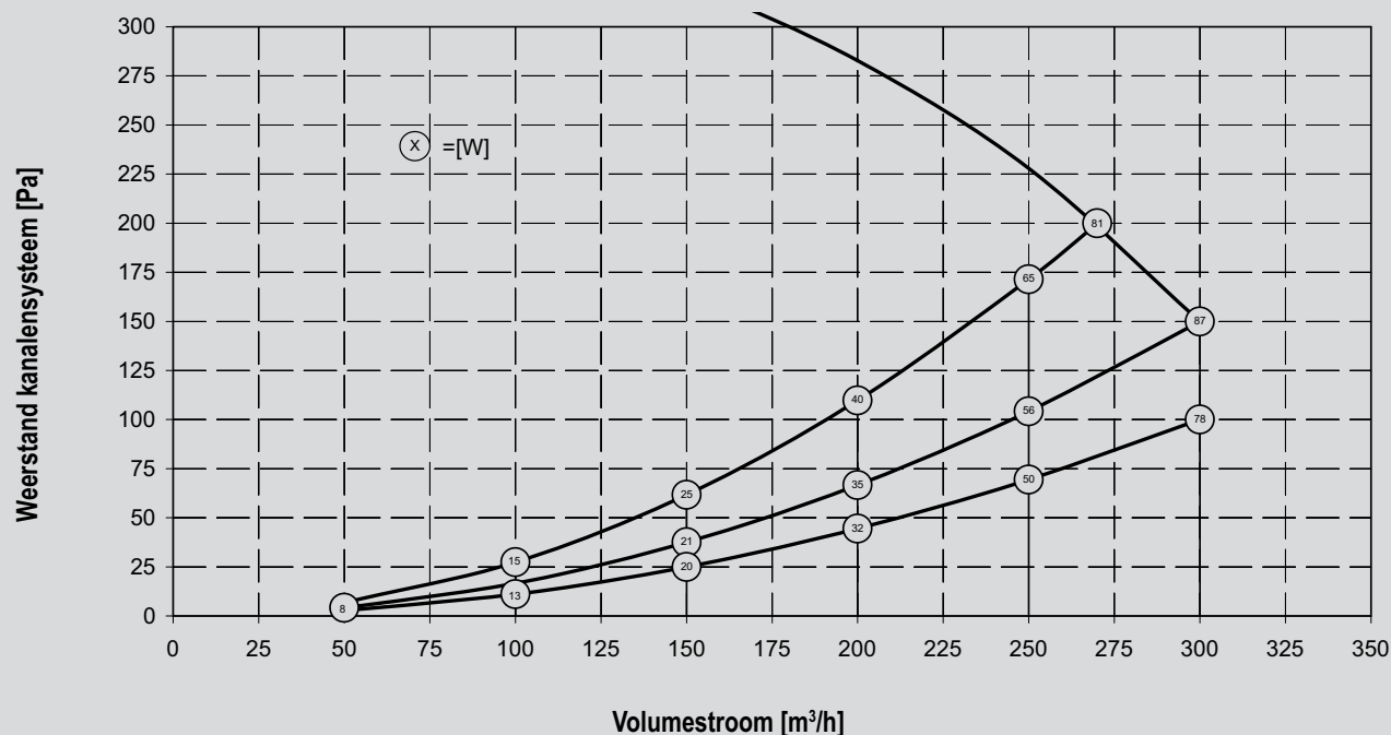
Ventilatorgrafiek Renovent HR Medium
