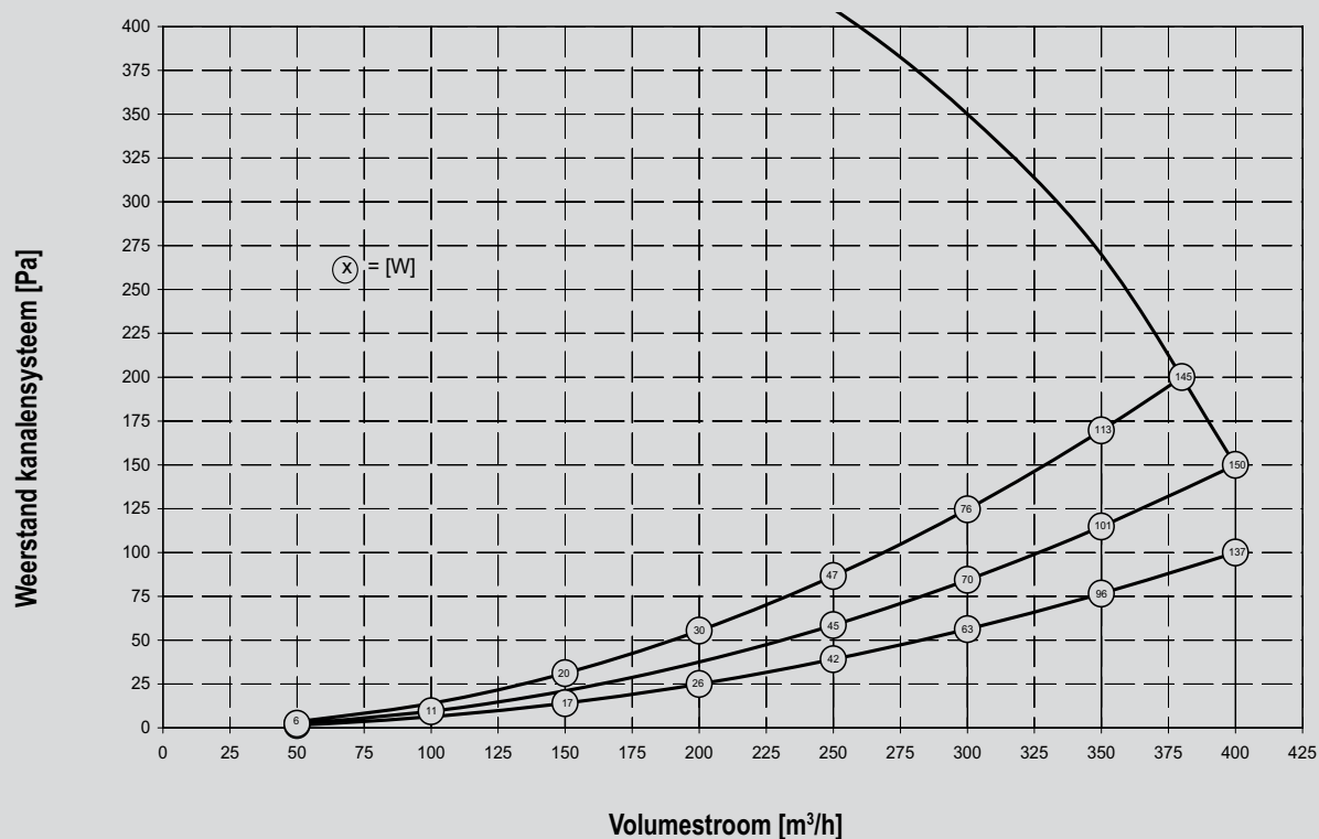
Ventilatorgrafiek Renovent HR Large
