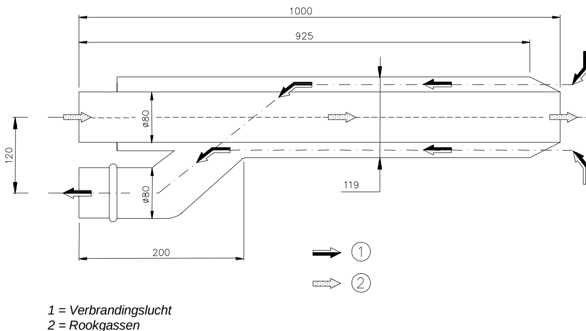
Figuur 6 : Horizontale geveldoorvoer ø80 SWB-toestel.
