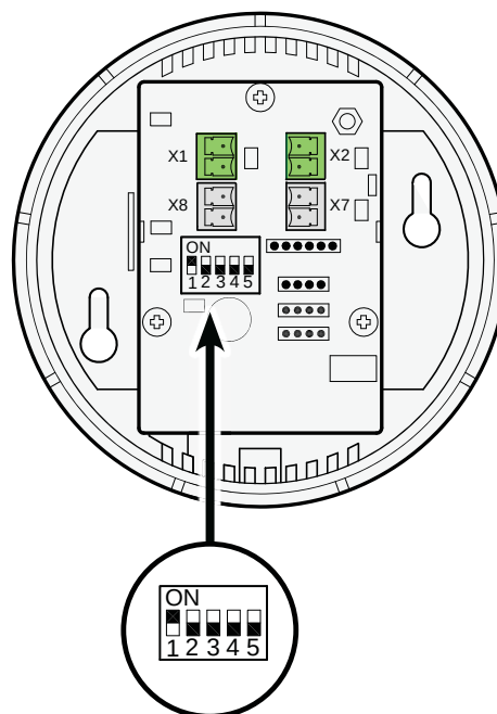
Exemple de réglage du CO 2 -sensor n°1
