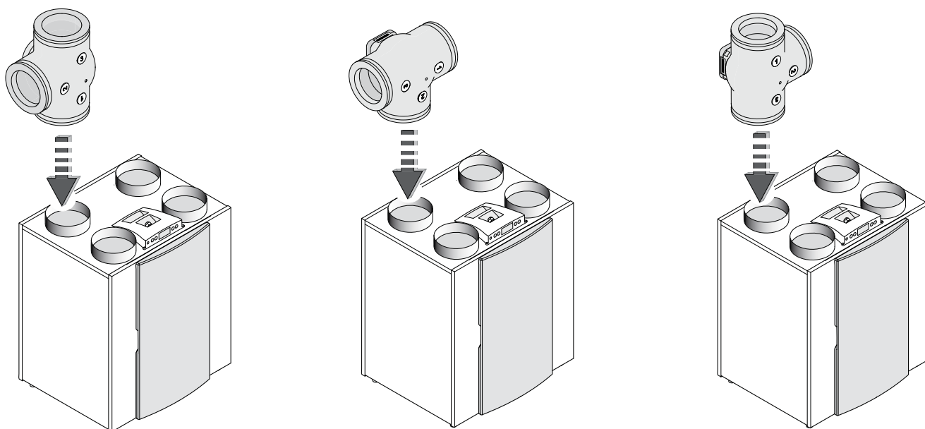
Exemples de raccord d'une soupape de zone sur le conduit d'apport d'air du récupérateur de chaleur
