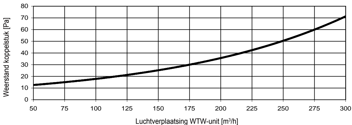
Figuur 6: Weerstand koppelstuk
