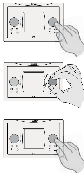
Figuur 5 Parameter CV+WTW activeren bij Renovent Sky
