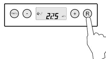
Figuur 4: Parameter CV+WTW activeren bij Renovent Excellent
